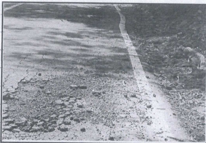
Foto 08 - Pista danificada com trincas tipo "jacaré" e trincas tipo "bloco"
